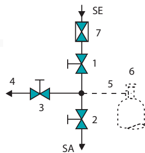
DPB 503 (3-Port-Version)
