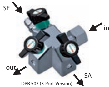
DPB 503 (3-Port-Version)
